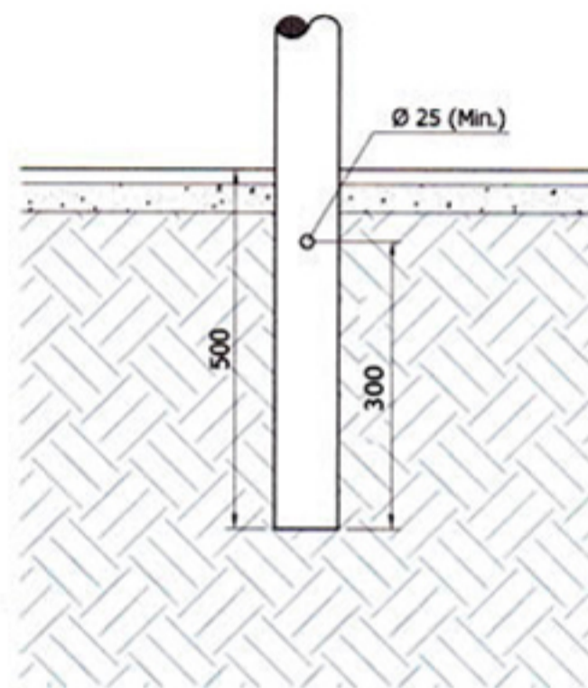
Detalhe de Engaste
